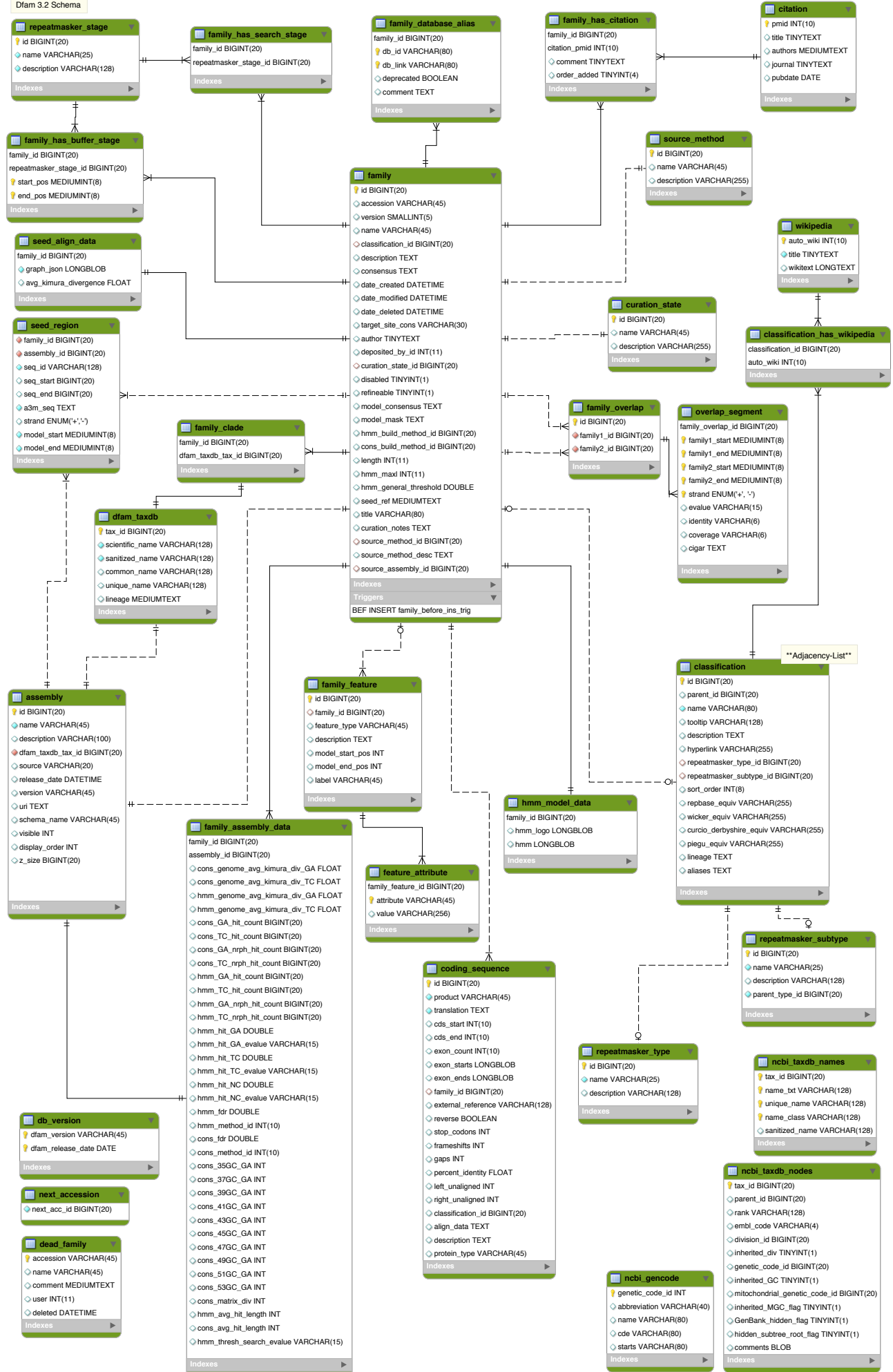
Dfam 3.2 Schema
